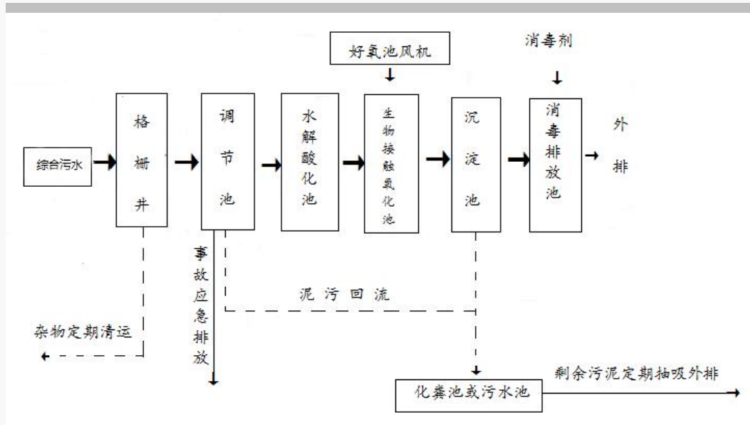
图3-3 污水处理工艺图
